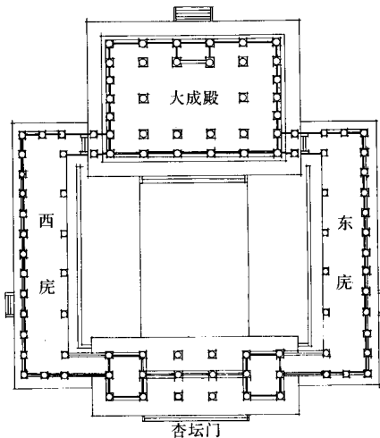
图1-13 日本汤岛圣堂殿庭平面图(《日本之建筑与艺术》)
