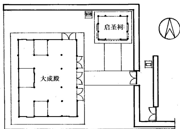
图 1—23 琉球首里孔子庙平面(《琉球建筑》)
