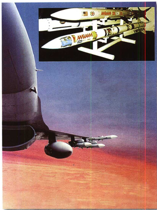
美国 AIM-120A “先进中程空空导弹” (AMRAAM)
