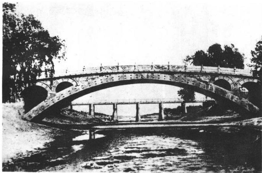
赵州桥(河北省赵县)
