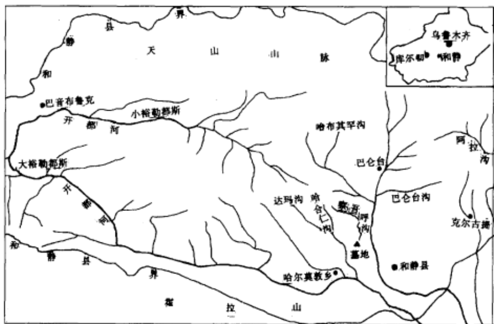
图一 察吾呼沟地理位置示意图
