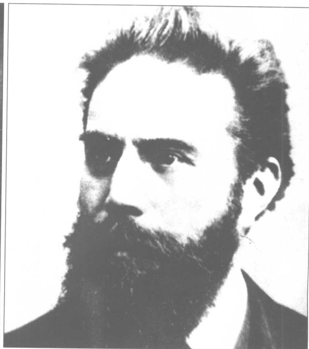
德国人威廉·伦琴因发明X光 线荣获第一届诺贝尔物理学奖。
