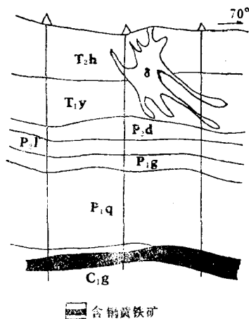
图 6 狮子山冬瓜山铜矿剖面示意图
