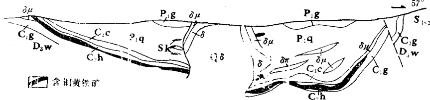
图 7 新桥铜矿纵剖面示意图
