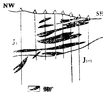
图 10 DPS 铜矿剖面示意图
