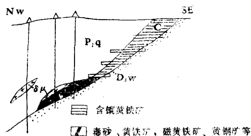
图4 铜官山松树山剖面示意图
