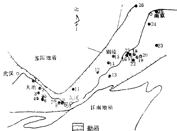
图1 长江中、下游大地构造分区及有关矿床分布略图
