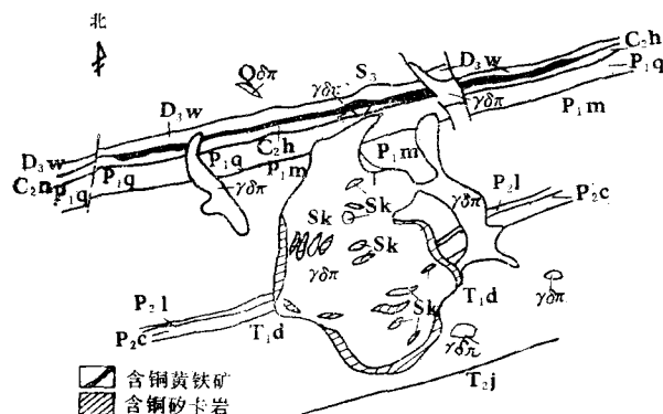
图2 武山铜矿平面示意图
