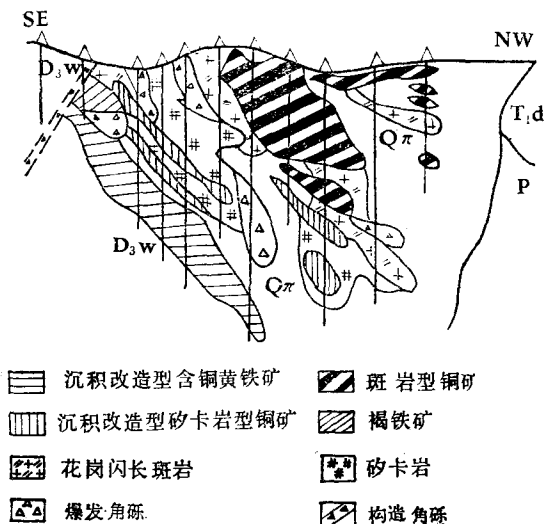
图3 城门山铜矿剖面示意图
