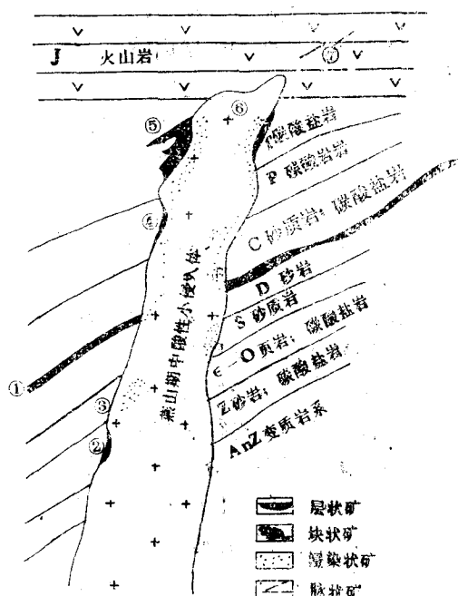
图 11 长江中、下游铜矿成矿复合模式图
