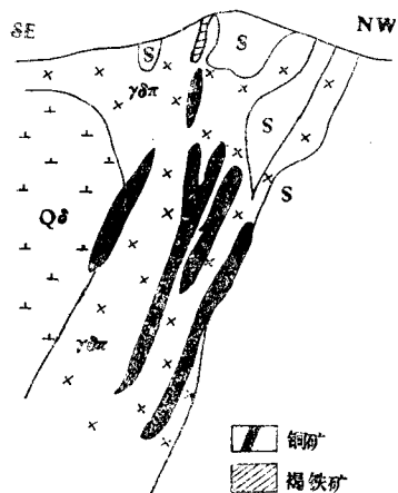
图 9 丁家山铜矿剖面示意图
