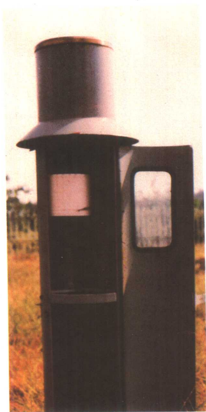
虹吸式雨量自记仪
