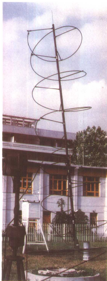
71型收讯机和118型传真收片机及天线
