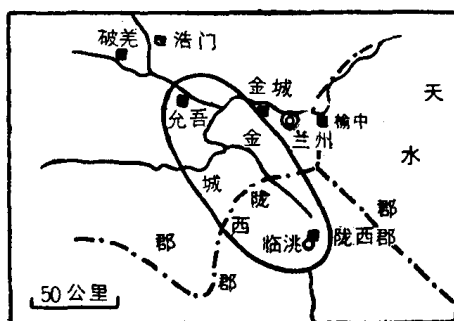
图4 138年金城、陇西地震震区图
