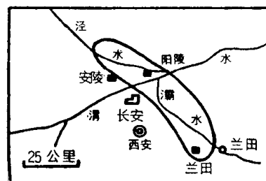
图3 前35年蓝田、咸阳地震震区图
