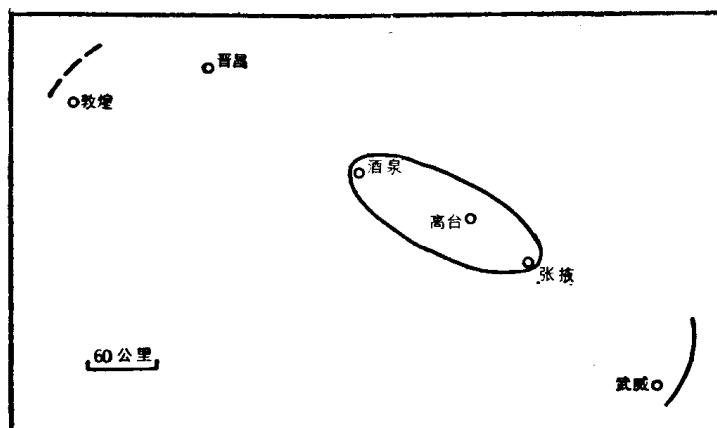
图7 756年河西地震震区图
