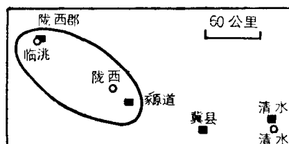
图2 前47年陇西地震震区图
