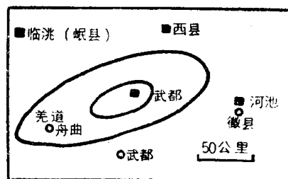
图1 前186年武都地震震区图
