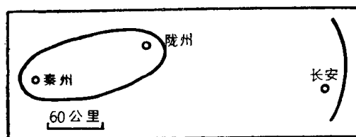
图6 600年秦陇地震破坏范围
