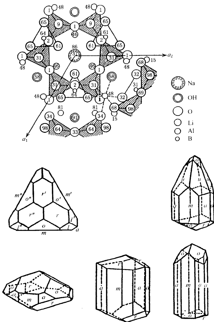
图 2-1 托玛琳的晶体结构
