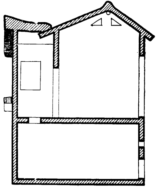
· 甲-甲 剖面图 ·
