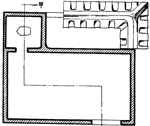
· 二层平面图 ·
