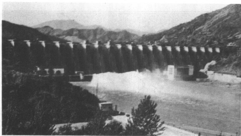
大别山水库群之一——佛子岭水库连拱坝
