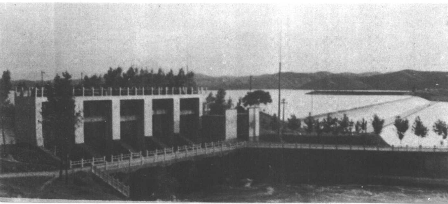
潞河总干渠的横排头渠首工程
