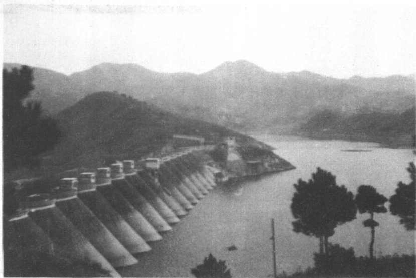
大别山水库群之一——梅山水库一角
