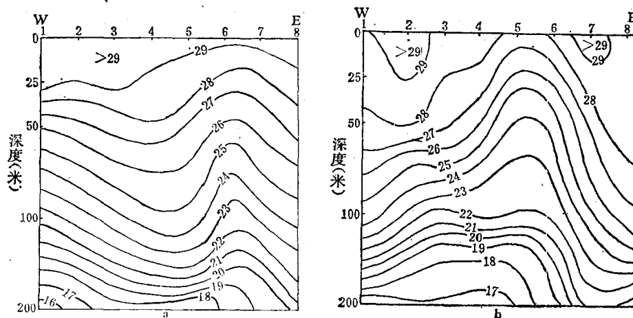
图4 鹅銮鼻以南的水温 T°C 断面
