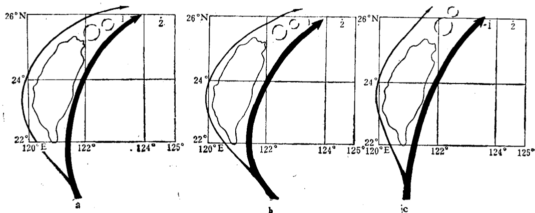
图 7 黑潮流绕台湾的简单模式 (图上以数字代表的地名, 1 钓鱼岛, 2 赤尾屿)
