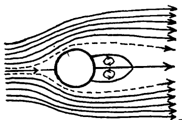
图 2 粘性流体流过圆柱体的模式(根据文献[4])
