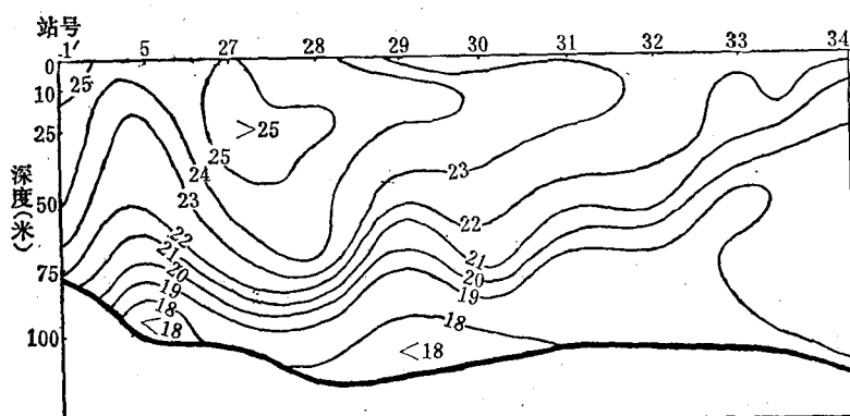
b. 1932年6月温度 T^{\circ}\text{C} 断面
