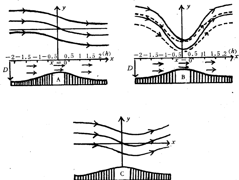
图8 海流跨越海脊时偏转的典型模式
