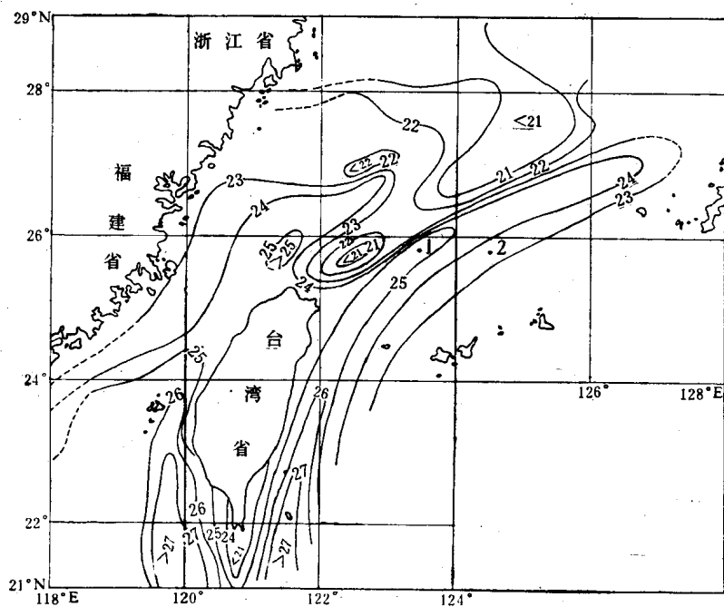
c. 50 米层, 1932 年 6 月上旬
