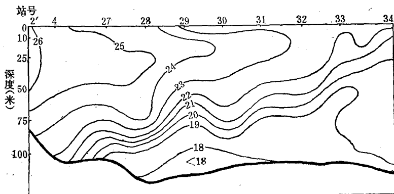
c. 1932年6月温度 T^{\circ}\text{C} 断面
