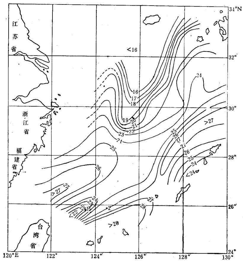
d. 50 米层, 1973 年 7 月 10 日—8 月 10 日
