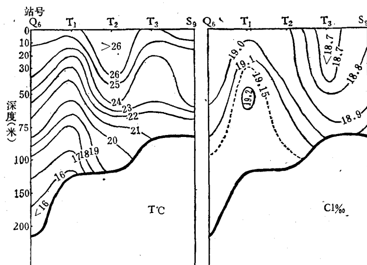
e. 基隆以北的纵向温、盐度断面, 1961年10月19—20日
