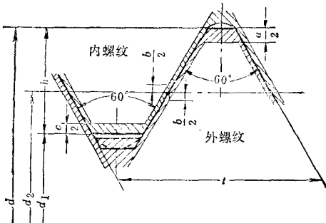
图 27·1-2 普通螺纹公差带位置
