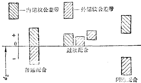
图 27-1-1 普通螺纹中径的公差与配合
