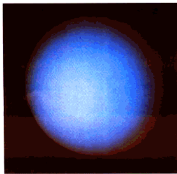
tiān wáng xīng 天王星
