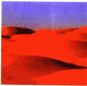
shā mǒ 沙漠
