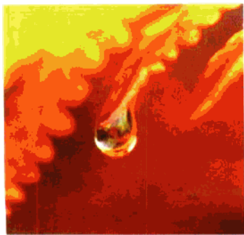
lù zhū 露 珠
