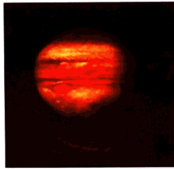
mù xīng 木星
