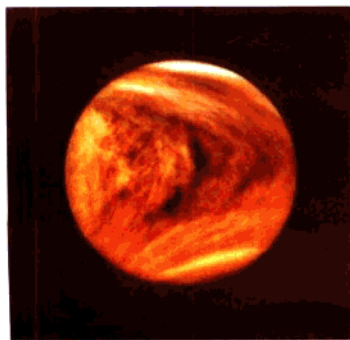
jīn xīng 金星
