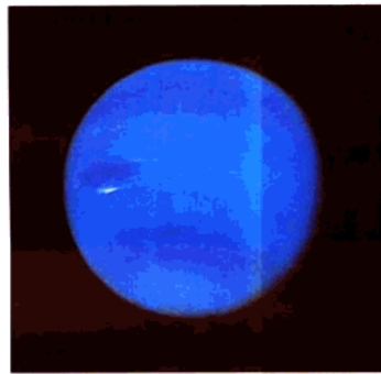
hǎi wáng xīng 海王星
