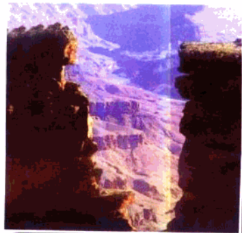
xiá gǔ 峡谷
