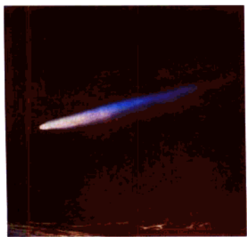
huì xīng 彗星
