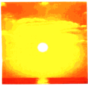
tài yáng 太 阳
