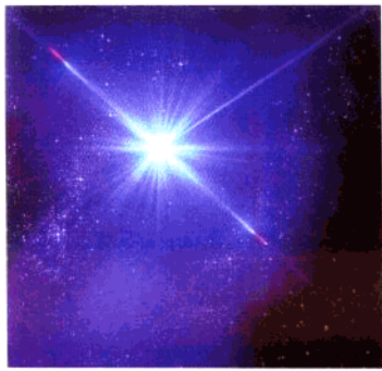
xīng xīng 星 星
