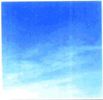
lán tiān 蓝 天
