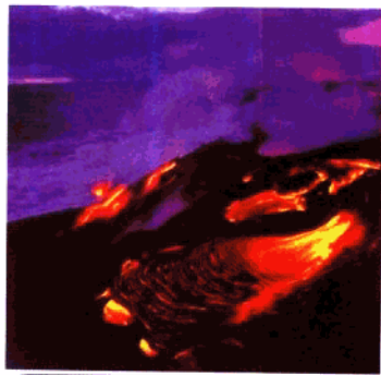
huǒ shān 火山
