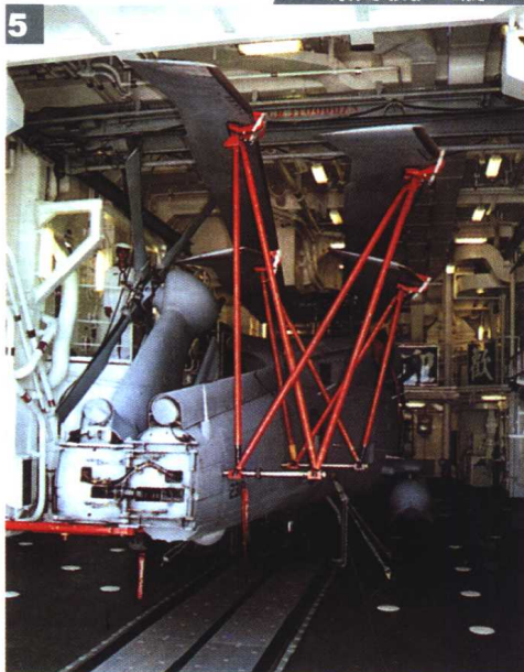
5. 康定级上的直升机库可容纳一架S-70C(M)-1型反潜直升机
