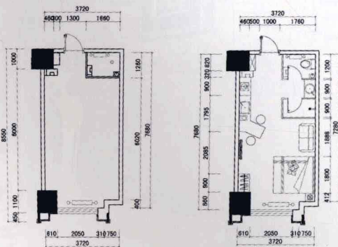
平面布置图
