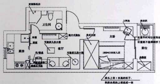
平面布置图
