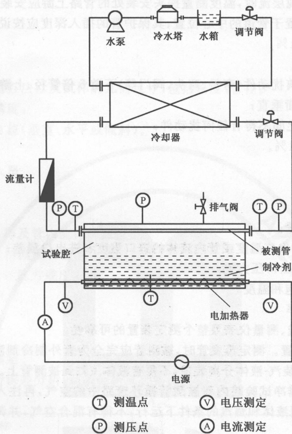
图 A.2 外冷凝管测定系统示意图
