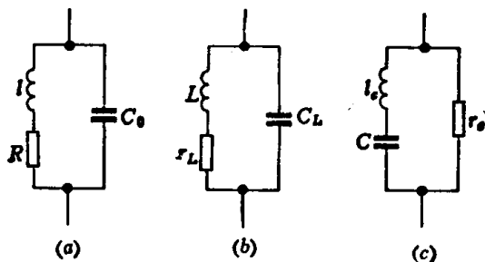
图2-1 元件等效电路图
