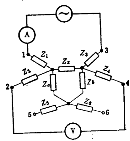
图2-3 四端测量的原理图
