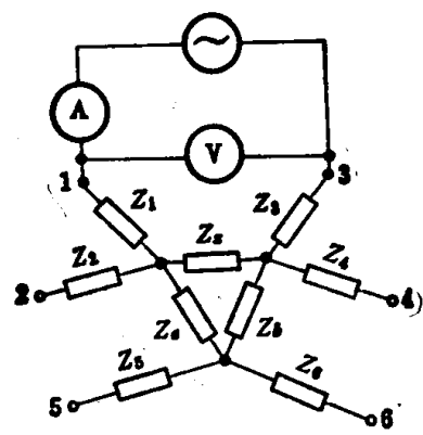
图2-2 二端测量原理图
