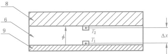
图 1 装有水冷散热片的热流计总装图
