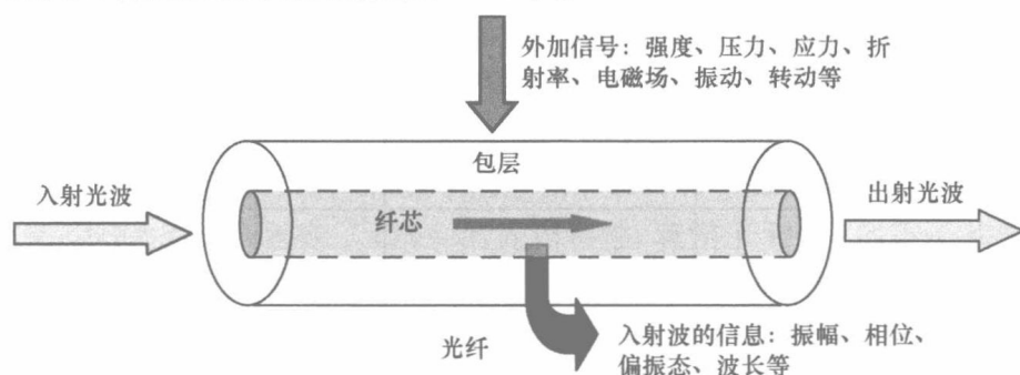
图 1-1 光纤传感原理
