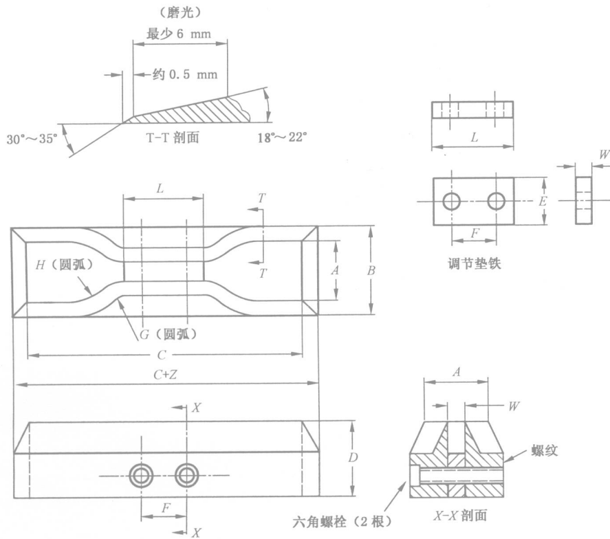
图 A.1 哑铃形试样模具图
