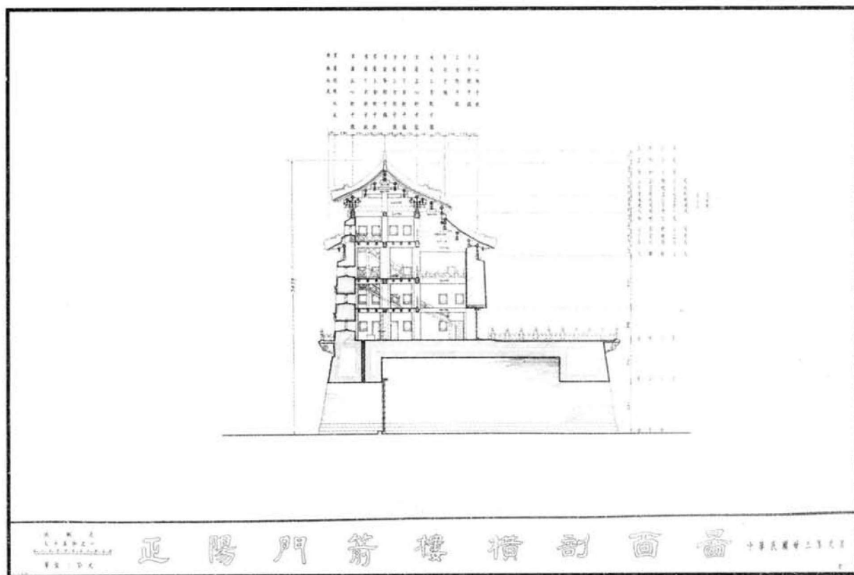
横剖面 1944年测图
