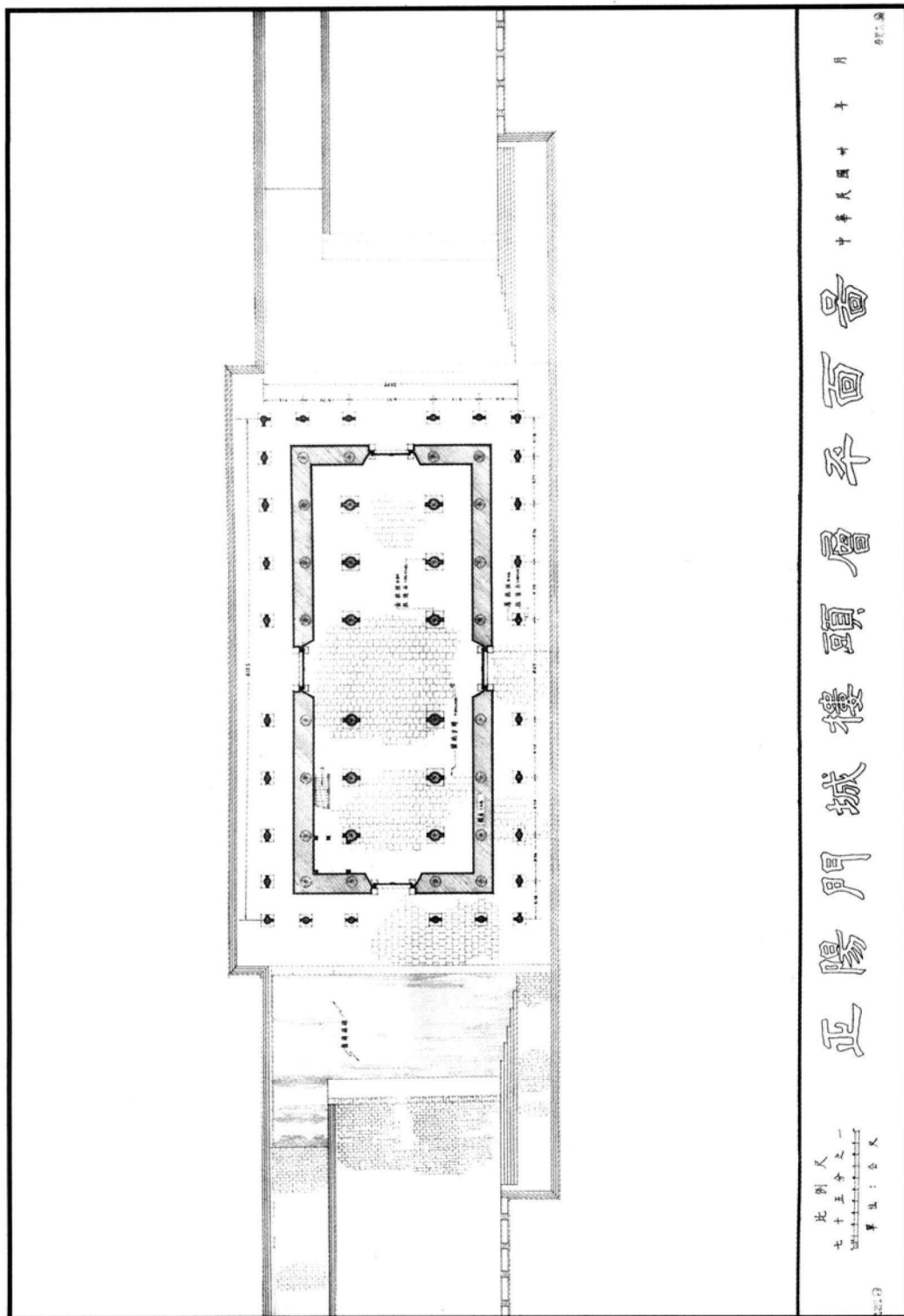
一层平面 1941年测图
