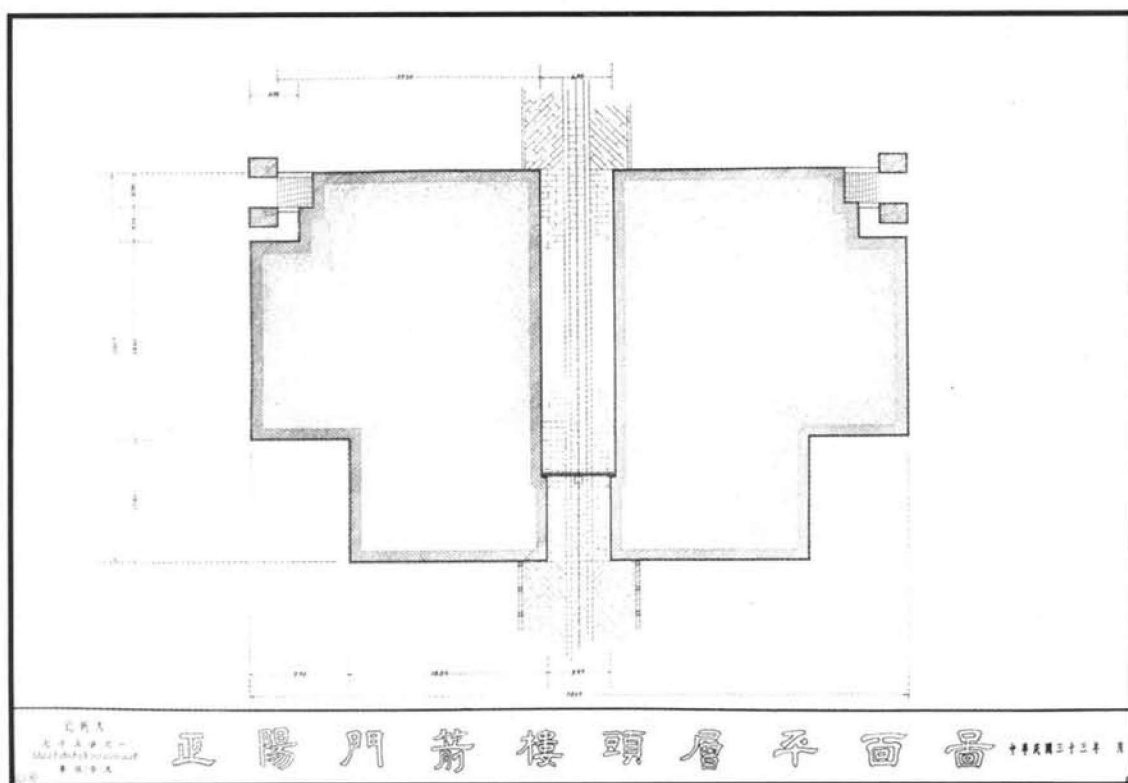
底层平面 1944年測圖
