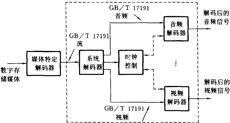
图 1 GB/T 17191 解码器样机原理图
