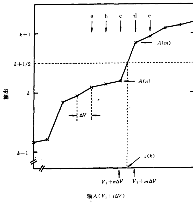
图 5A 直流电压校准
