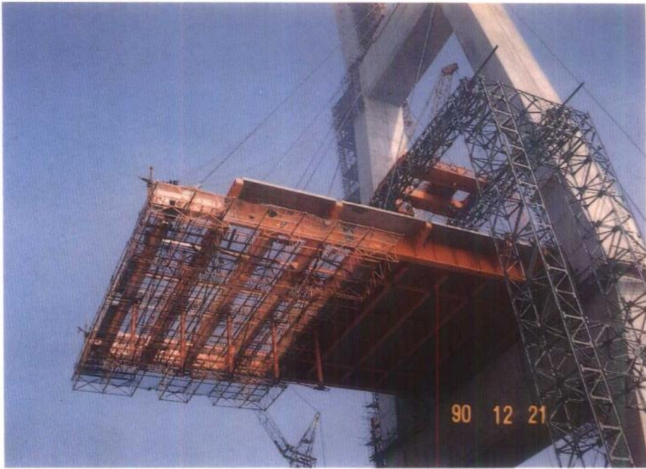
图8-97 南浦大桥钢梁拼装
