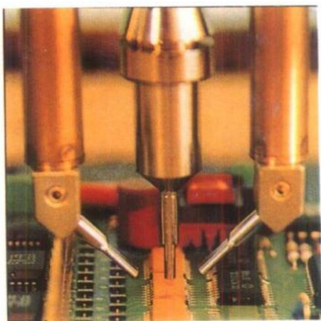
图11-24 热氮再流软钎接
