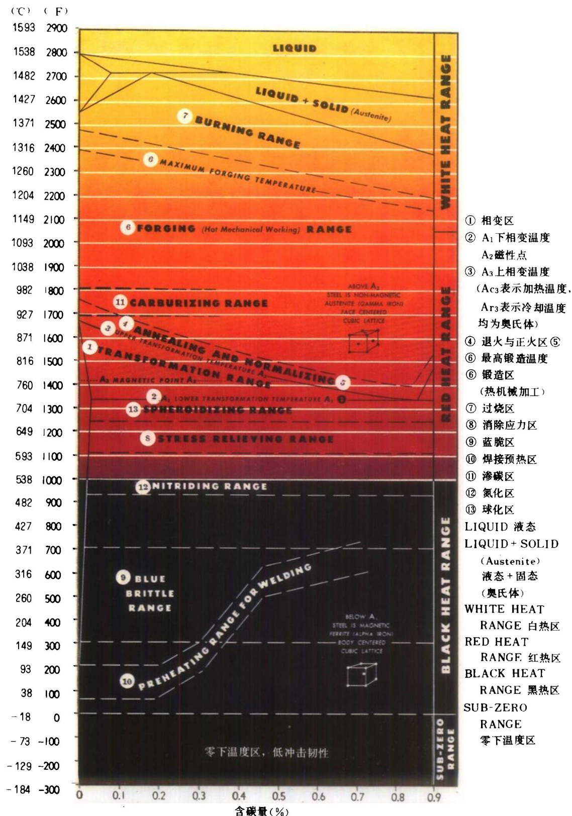
图1-1 C \leq 0.9\% 碳素钢从液态到零下温度的颜色变化
