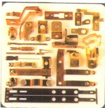
图11-59 现代继电器的 银触点
