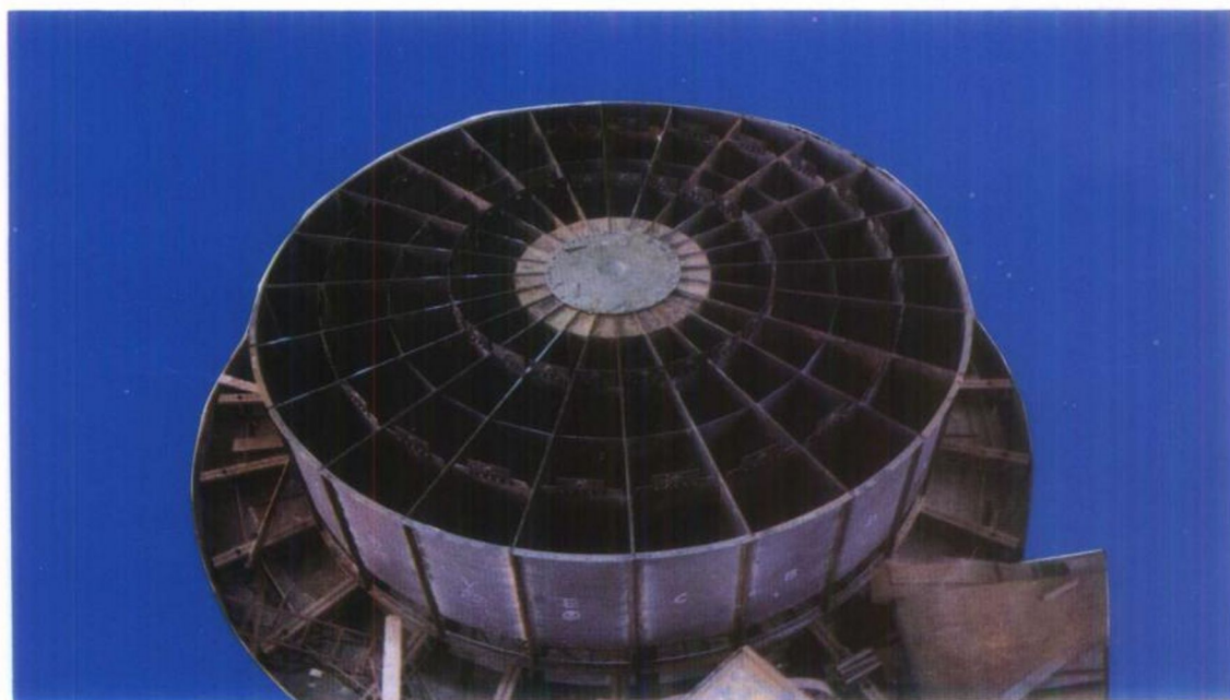
制造完成的30万千瓦预热器转子
