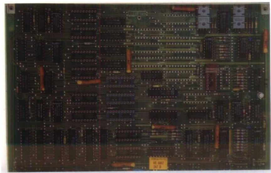
图11-52 六层印刷电路 板大面积无损 拆卸前的外观
