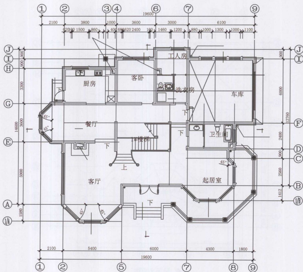
◆ 一层平面图
