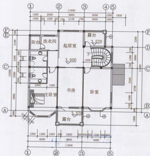
◆ 二层平面图
