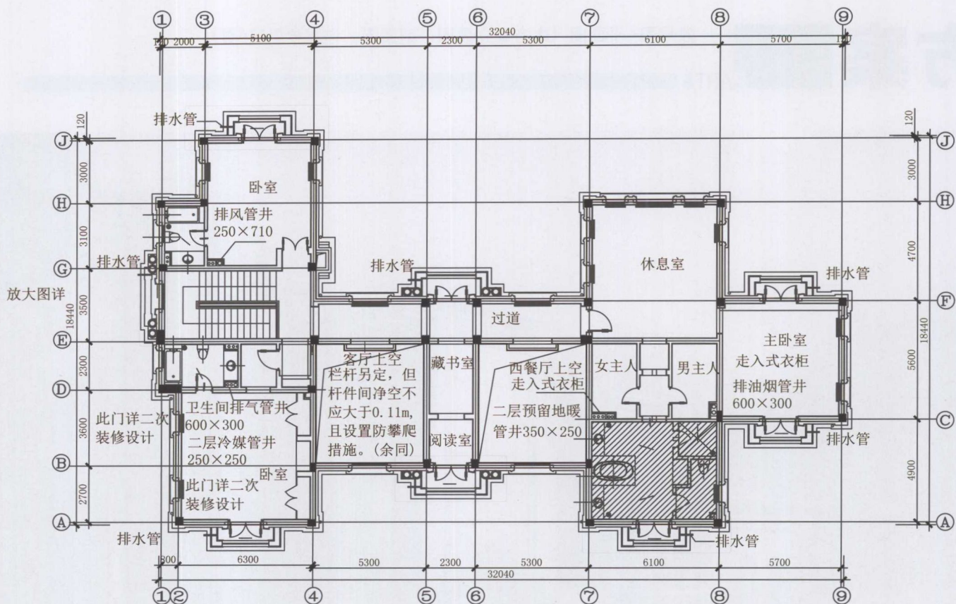
◆ 二层平面图
