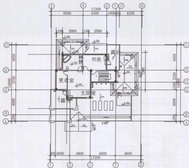
◆ 三层平面图
