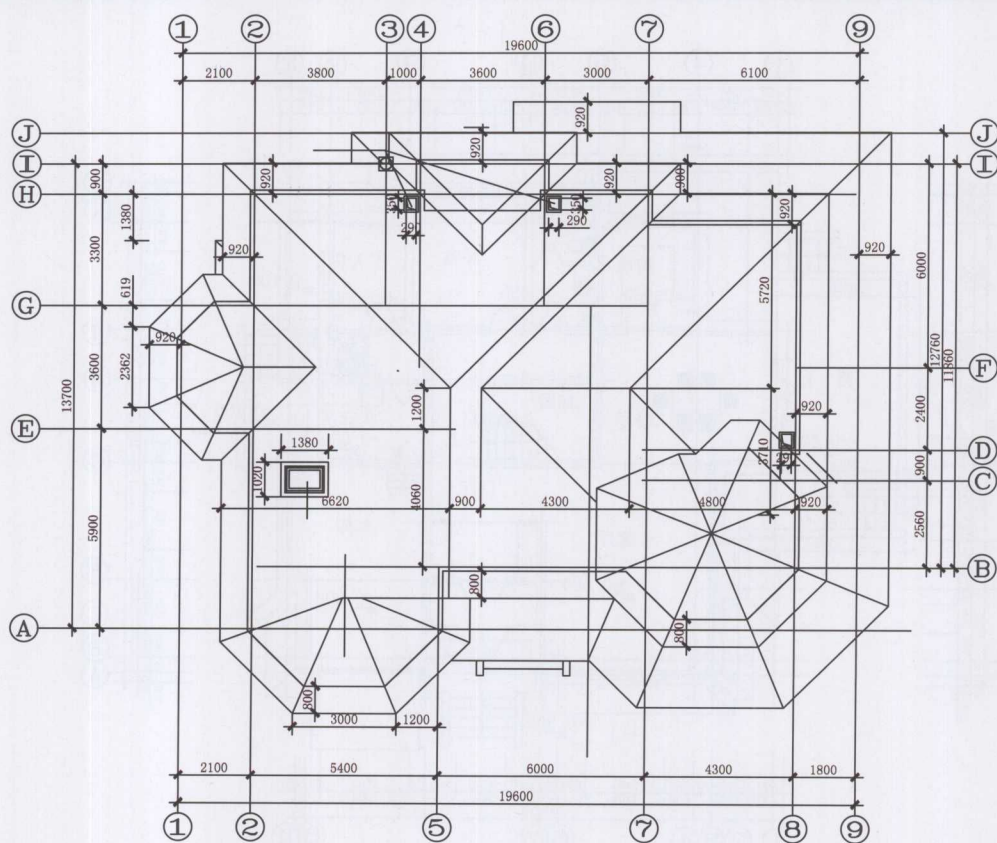
◆ 屋顶平面图
