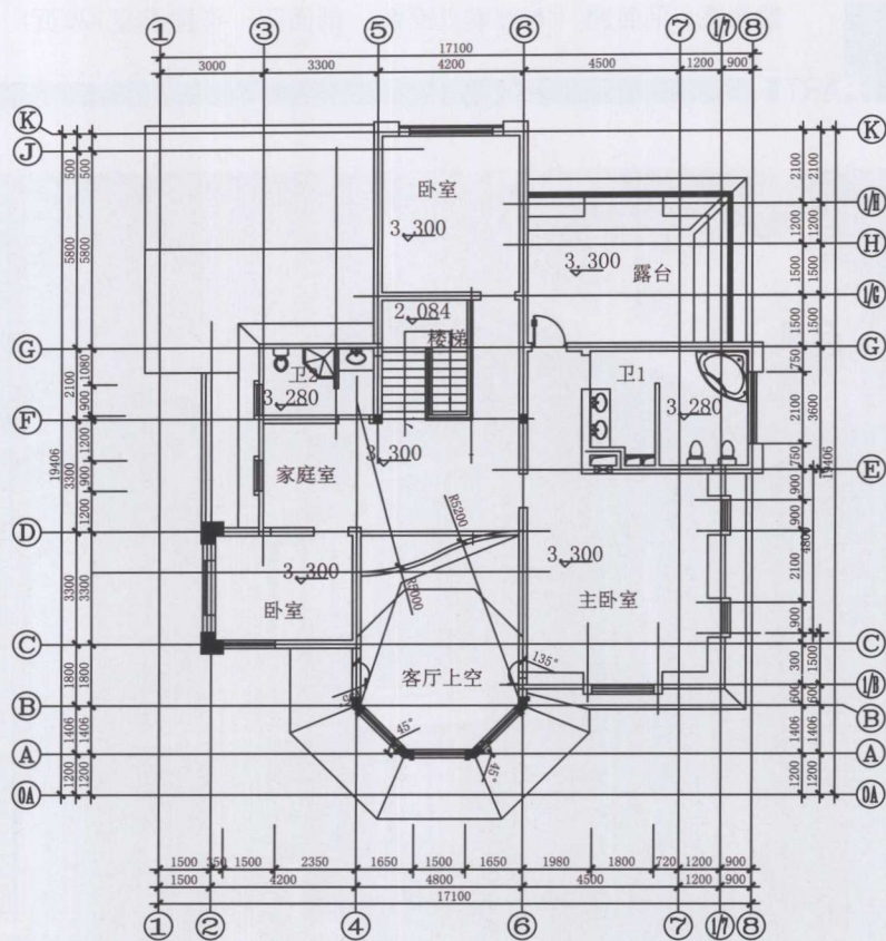
◆ 二层平面图
