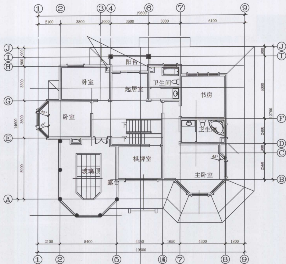
◆ 二层平面图
