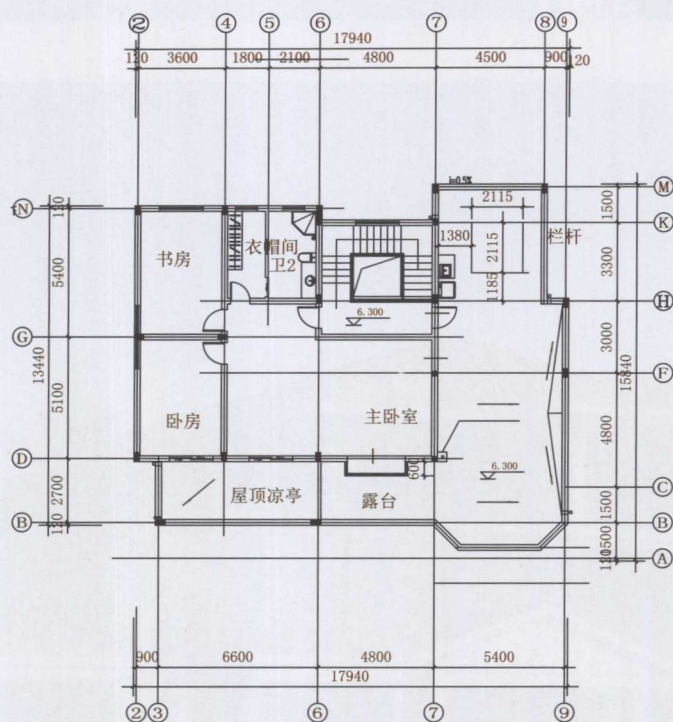
◆ 三层平面图
