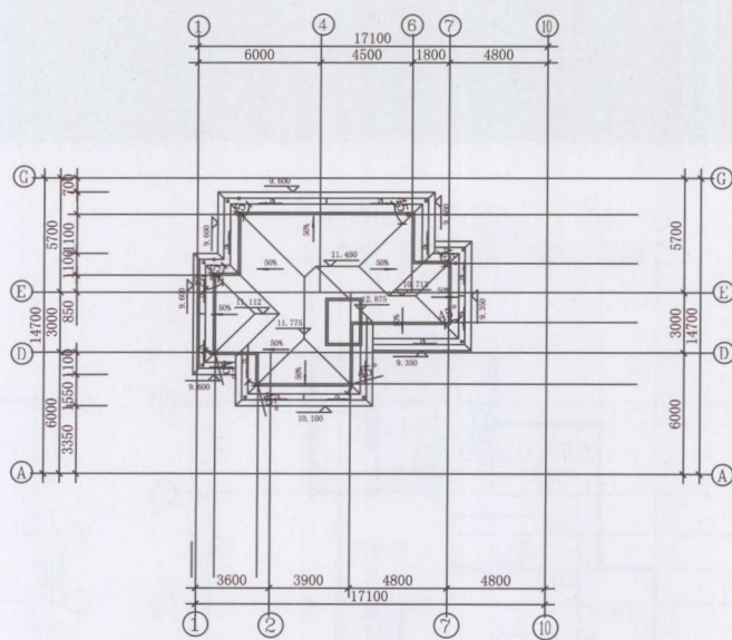
◆ 屋顶平面图
