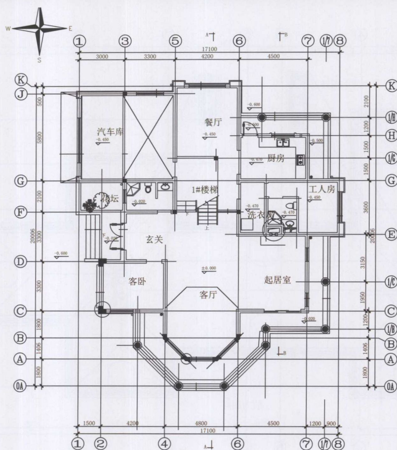
◆ 一层平面图
