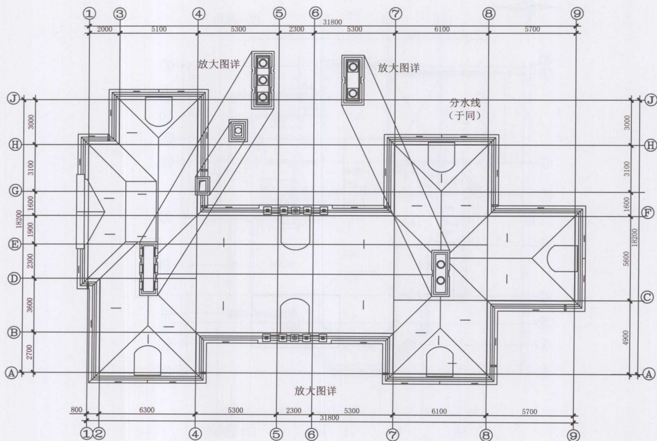
◆ 屋顶平面图
