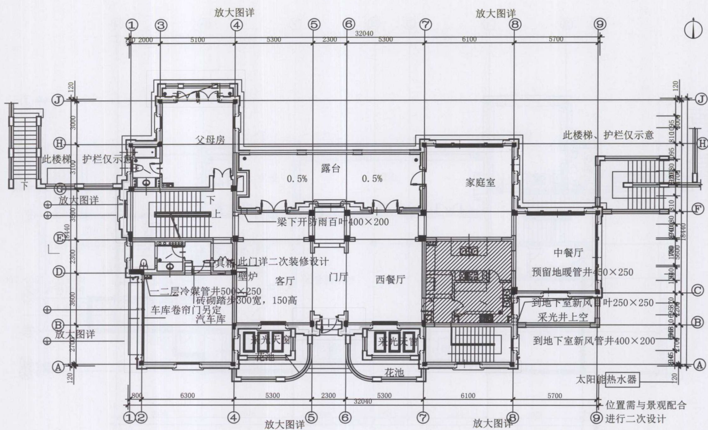
◆ 一层平面图
