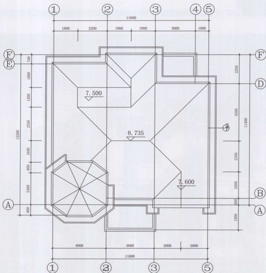
◆ 屋顶平面图
