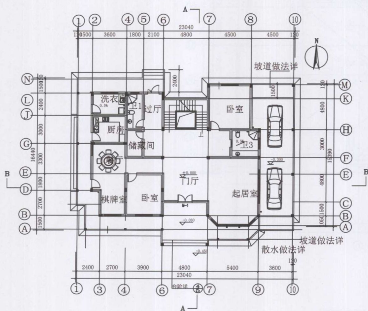
◆ 一层平面图
