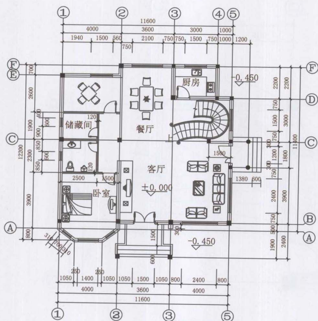
◆ 一层平面图
