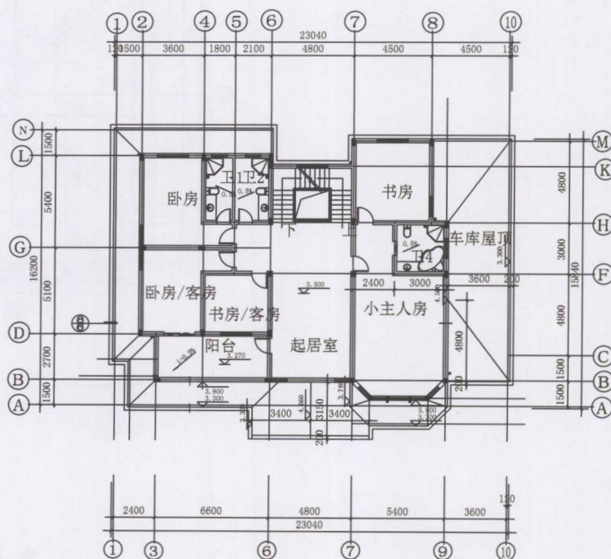
◆ 二层平面图
