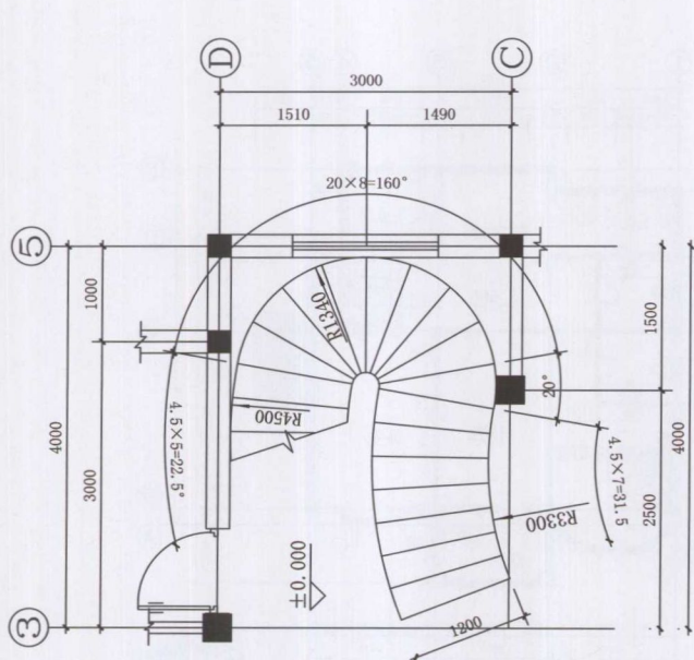
◆ 一层平面图
