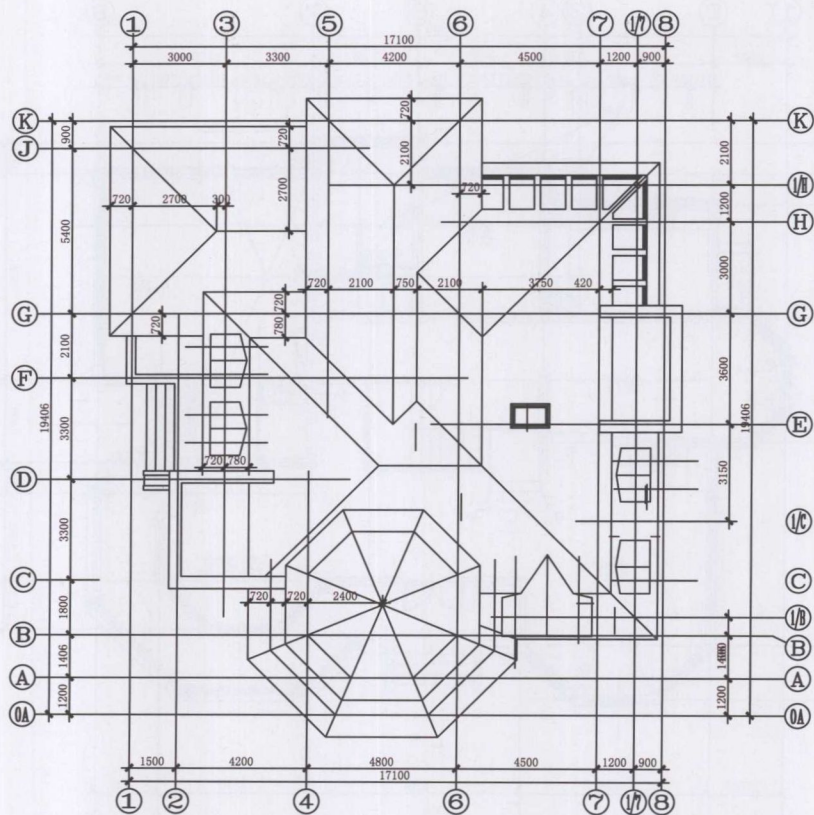
◆ 屋顶平面图
