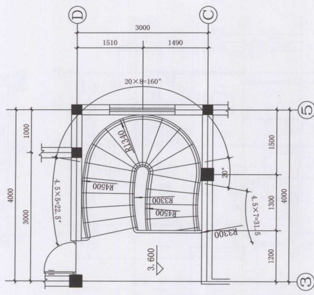
◆ 二层平面图
