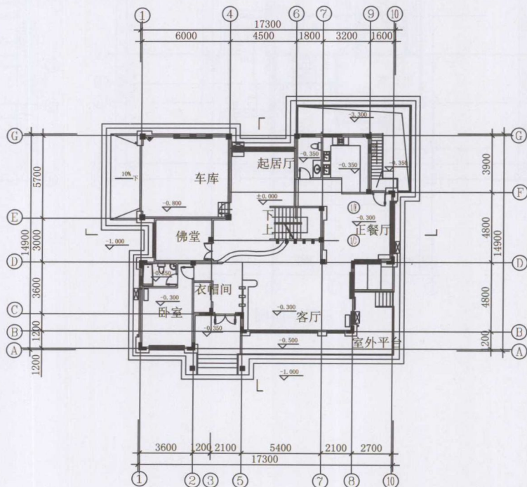
◆ 一层平面图
