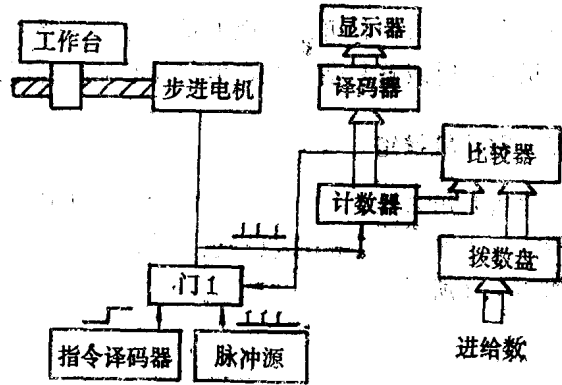
图 1.3 简易数控机床
