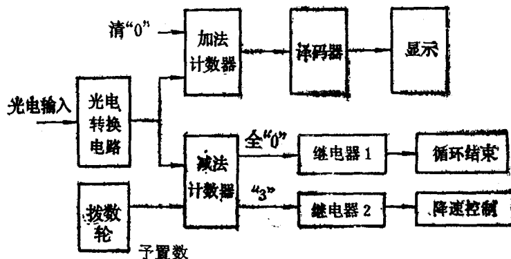
图 1.2 数片机线路框图
