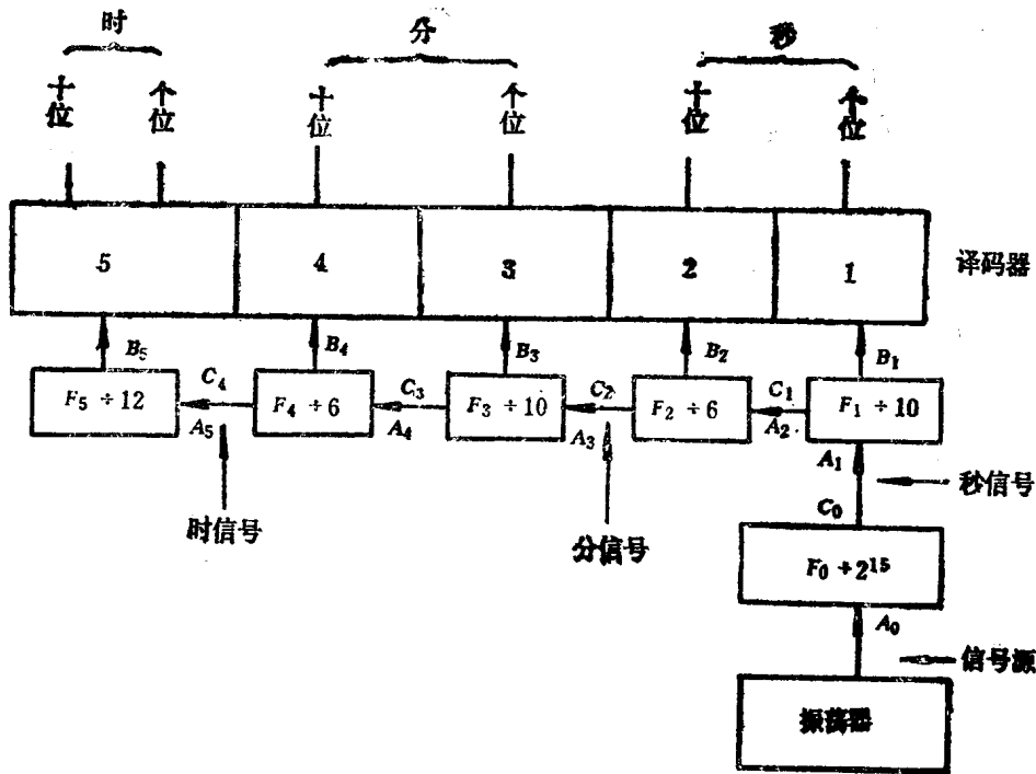
图 1.1 计时线路方框图
