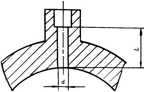
取压孔示意图
