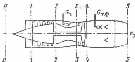
图1.1 涡轮喷气发动机示意图
