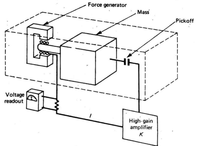
Fig. 3. Simple servoed accelerometer.
