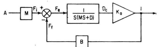
Fig. 3. Simple servoed accelerometer.
