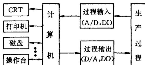
图 1.4 直接数字控制系统框图
