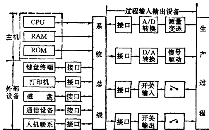
图 1.2 过程计算机控制系统的硬件组成框图
