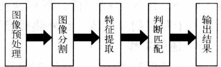
图 1-8 图像识别系统框图
