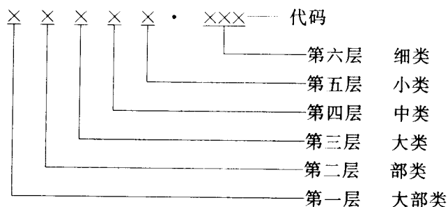
图 1 代码结构
