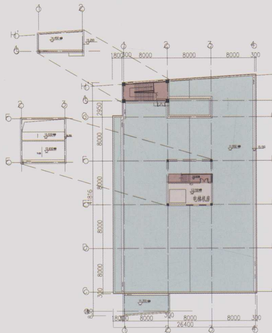
A 区体检中心屋面平面图
