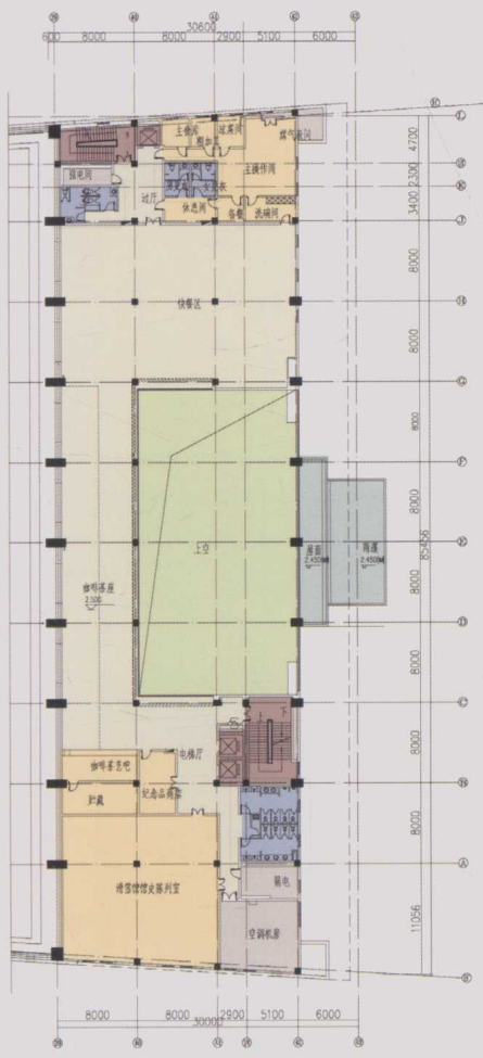
D区服务区二层平面图
