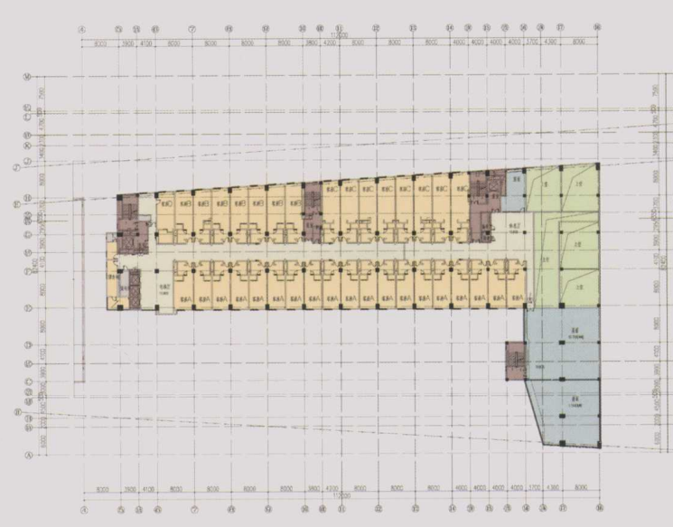
B区配套区三层平面图
