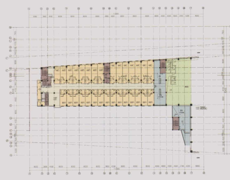
B区配套区五层平面图
