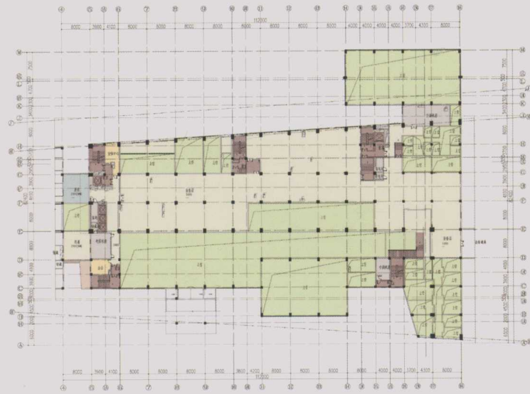
B区配套区夹层平面图
