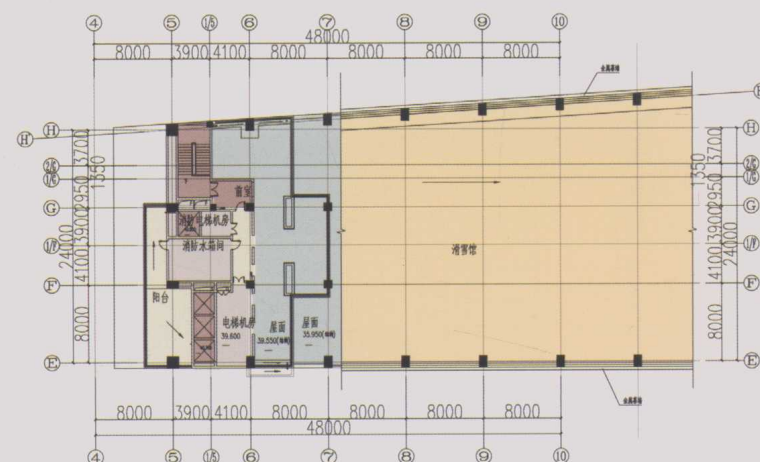
B 区配套区十一层平面图
