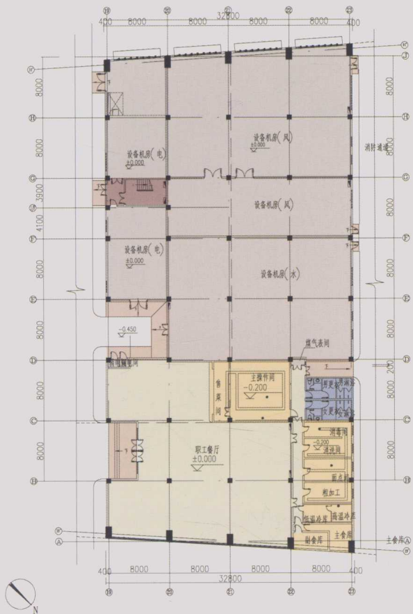
C区设备机房区一层平面图
