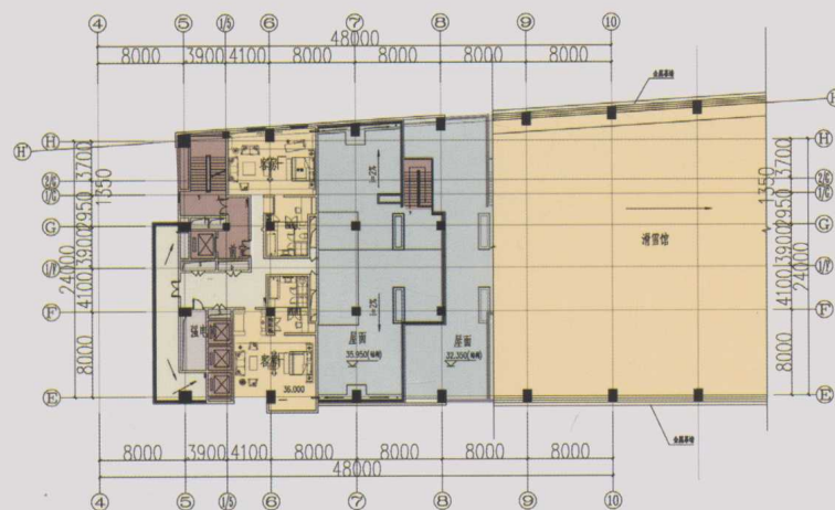
B 区配套区十层平面图
