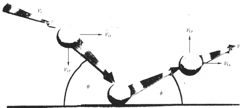
图7 网球反弹矢量示意图
