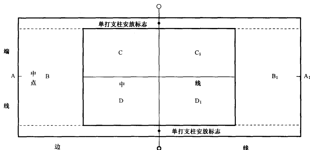
图 3 平整度检测点位示意图
