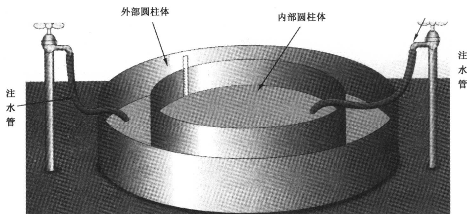
图 8 场地面层渗水性测定装置示意图
