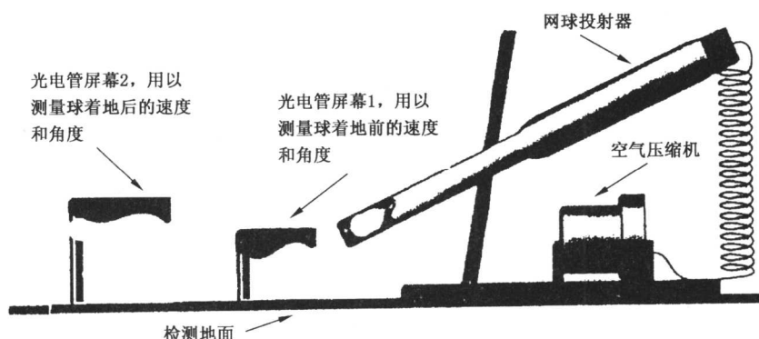
图 6 地面速率检测装置
