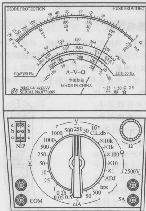
图 1-6 MF-47 型万用表的面板示意图
