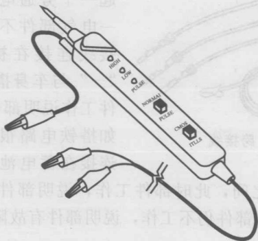
图 1-3 逻辑检测仪
