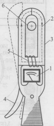
图 1-5 钳形电流表的结构原理
