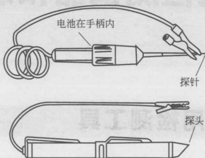
图 1-2 自带电源测试灯
