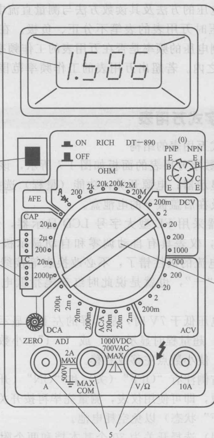
图 1-7 DT-890 型数字万用表
