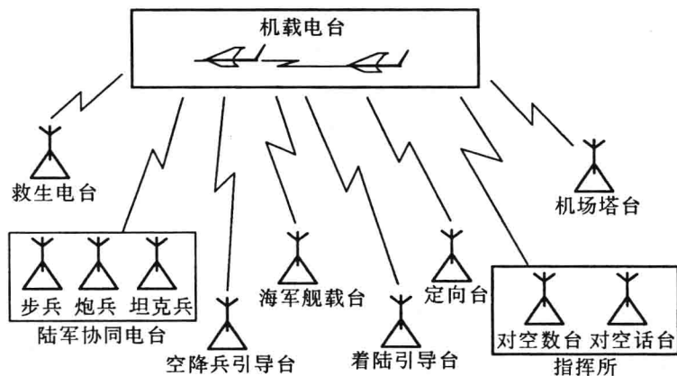
图 2-2 空军地 - 空通信系统示意图
