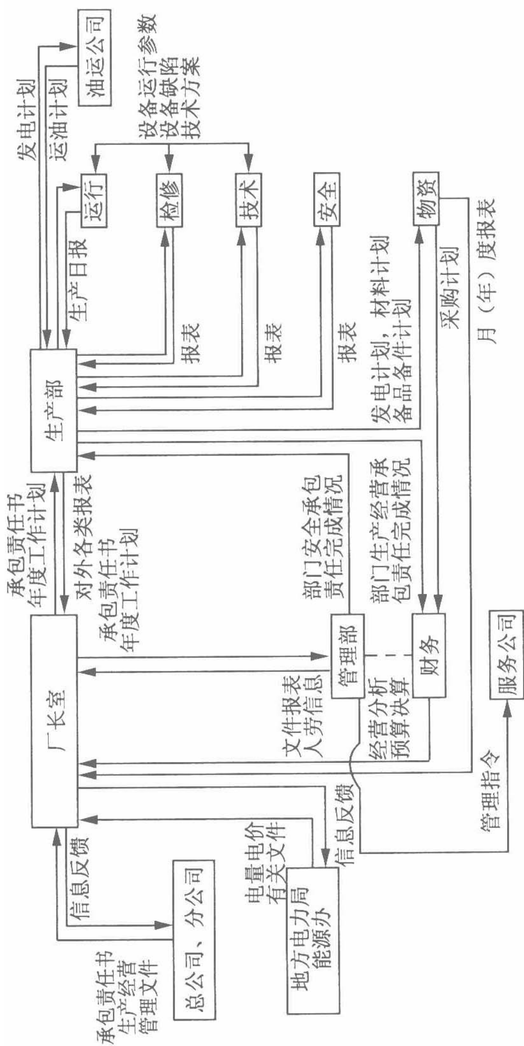
图3 汕头燃机电厂信息流图
