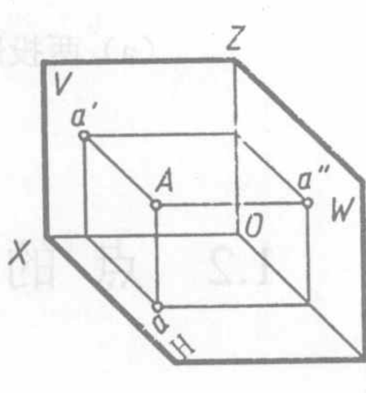
(a) 直观图
