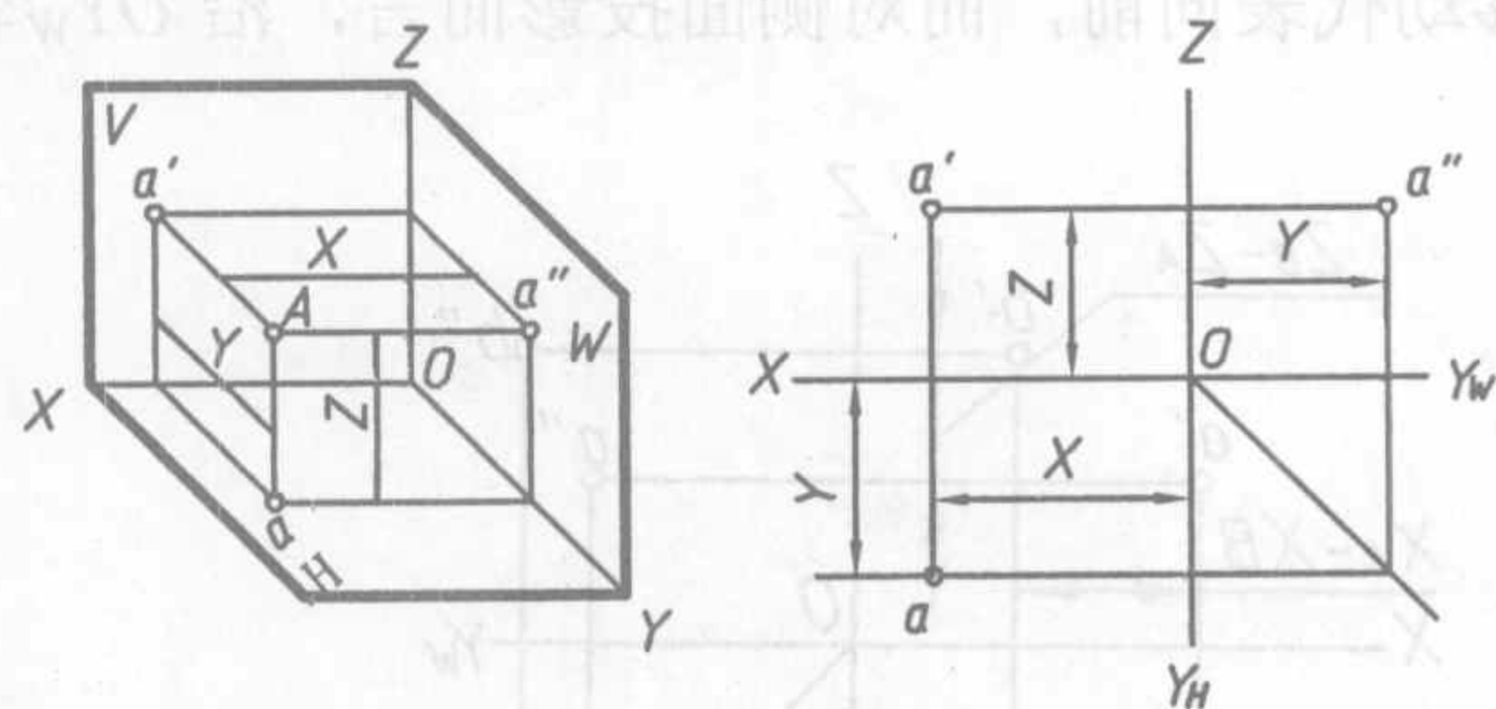
(a) 直观图
