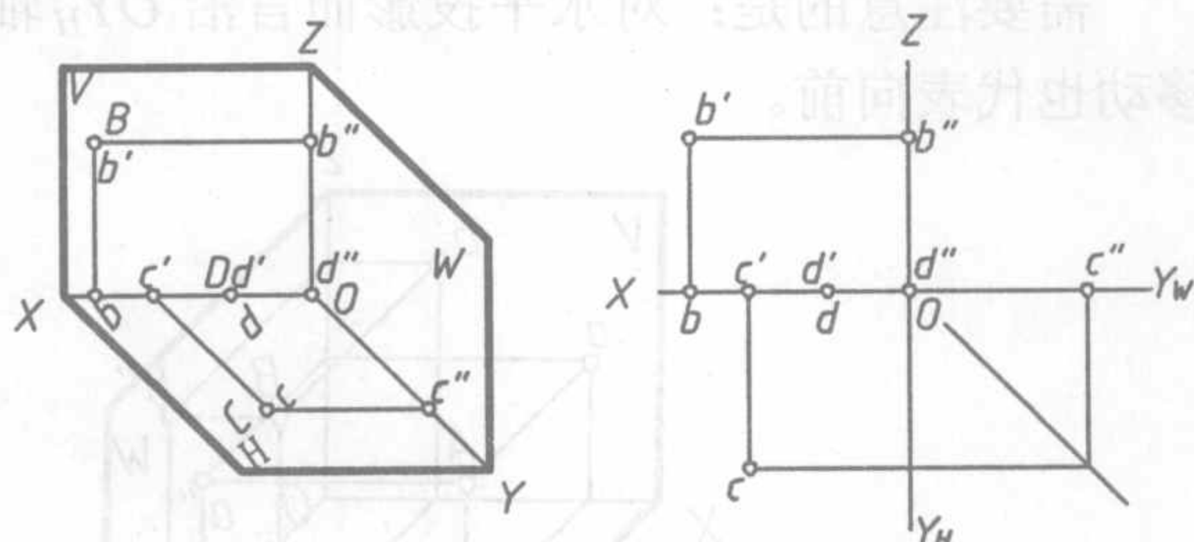
(a) 直观图
