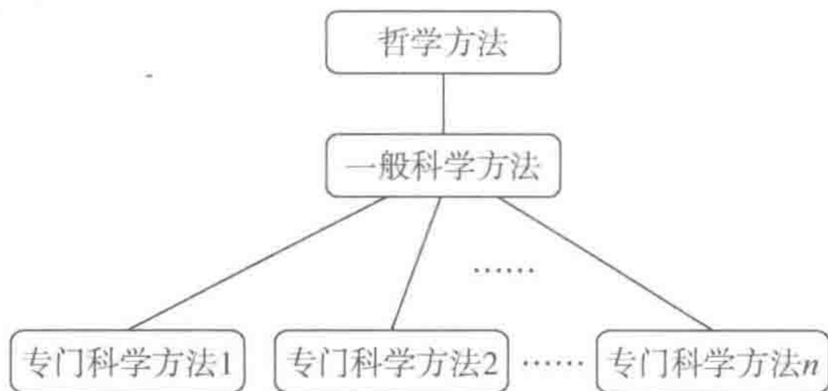
图 1-1 科学方法三层次
