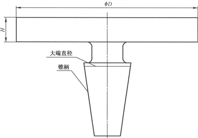
图 A. 2 检验圆盘
