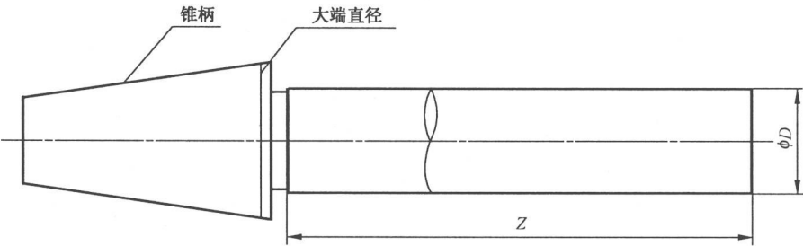
图 A. 1 检验芯轴
