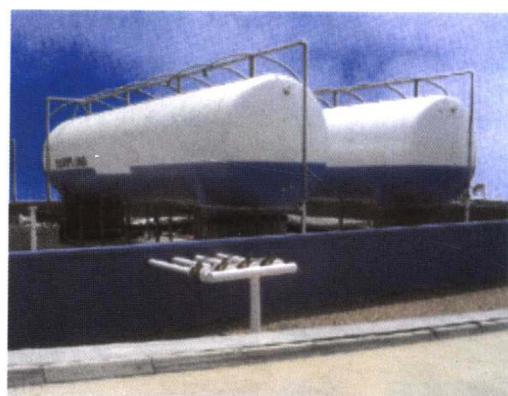
④LNG 气站卧式低温储罐
