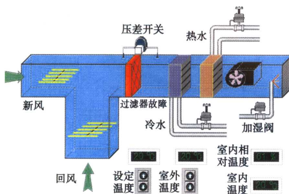
⑩空调箱系统工作过程仿真
