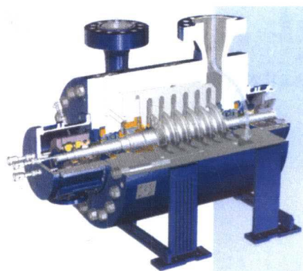
③离心式制冷压缩机的内部构造
