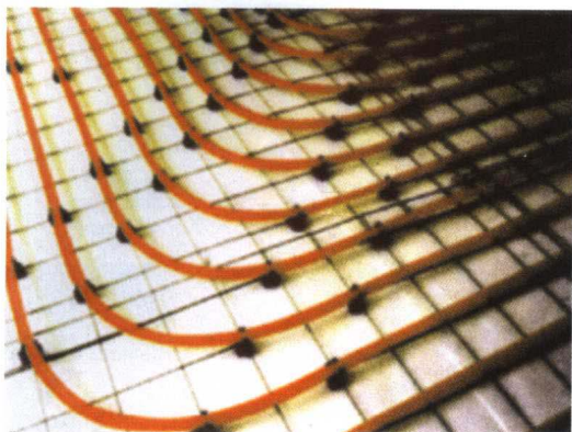
①预埋于活动地板下的辐射供暖系统管路
