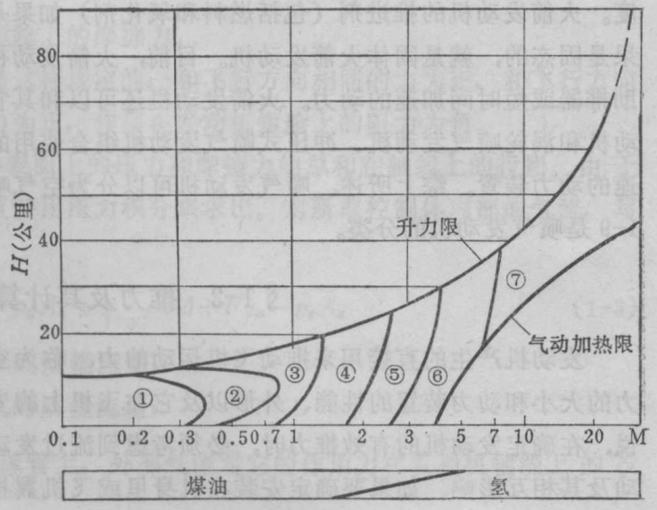
图 1-8 空气喷气发动机应用范围
