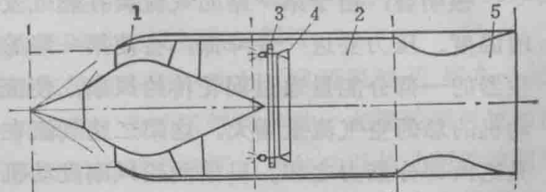
图1-7 超音速冲压式喷气发动机示意图
