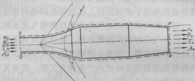
图 1-11 推导推力公式用图
