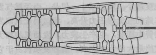
图1-6 涡轮轴发动机示意图
