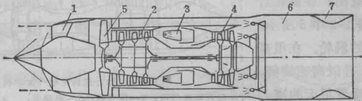
图1-4 加力式涡轮风扇发动机示意图
