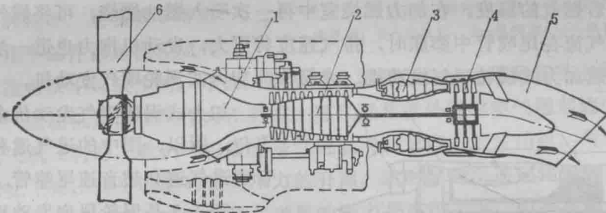
图1-5 涡轮螺旋桨发动机示意图
