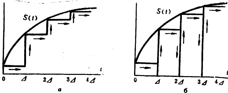
图 1.3 信号的动态表示法 (箭头表示每个基本单元随时间变化的路线)
