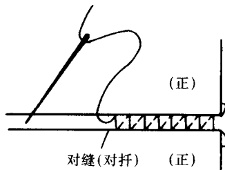
图 1-1-11 对缝
