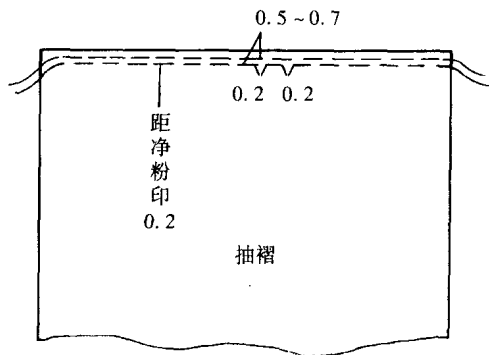
图 1-1-1(3) 抽褶
