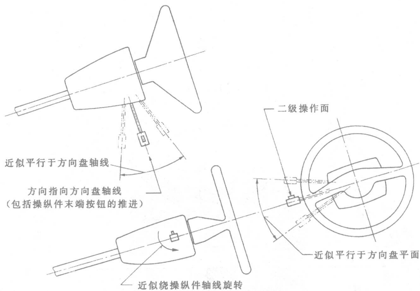
图4 操纵杆操作模式
