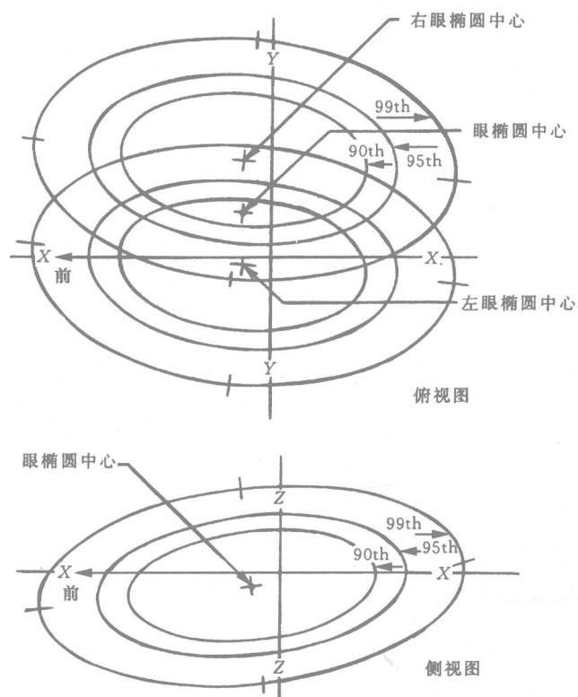
图 A1 H 点行程为 140 的眼椭圆
