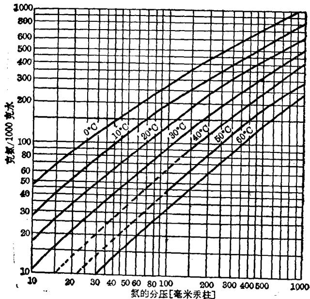
图 5-3 氨在水中的溶解度
