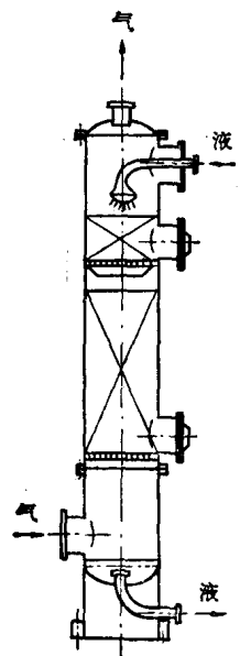
图 5-2 填料塔示意图
