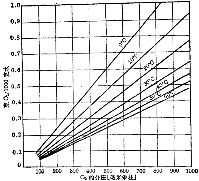
图 5-5 氧在水中的溶解度
