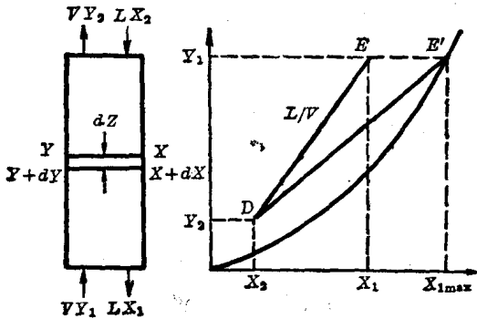
图 5-6 逆流操作填料吸收塔的物质衡算
