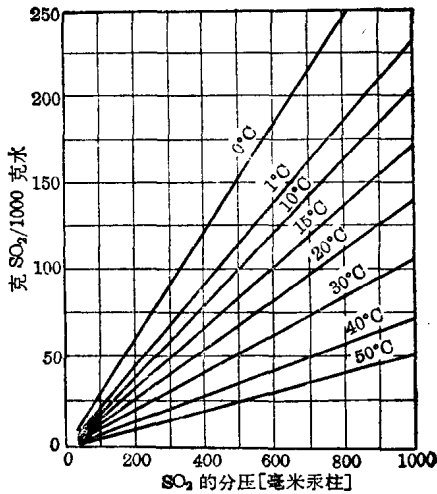
图 5-4 二氧化硫在水中的溶解度
