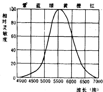
图 1-1 视觉相对灵敏度与波长的关系
