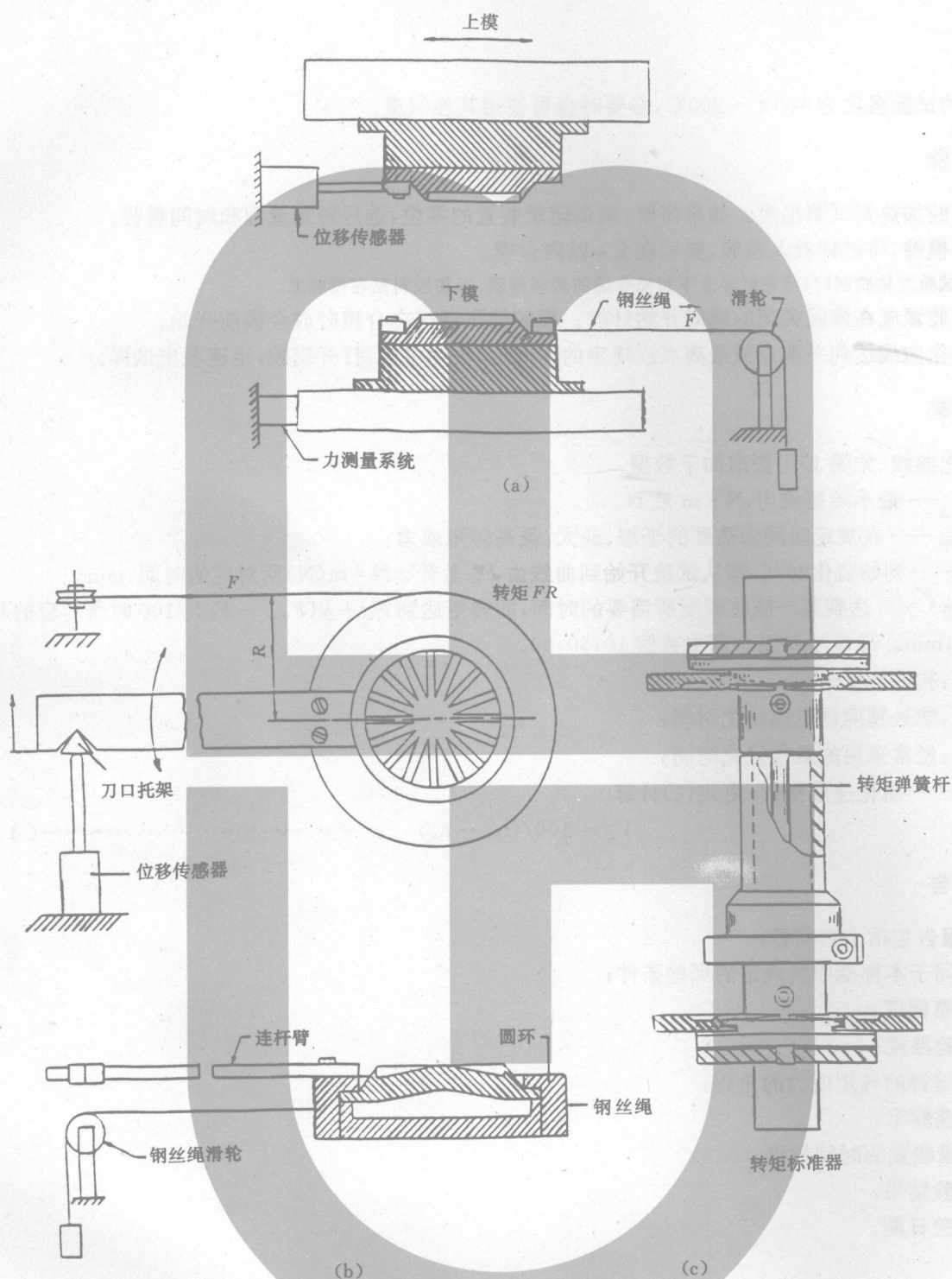
图 3 对应的三种硫化仪的校正装置
