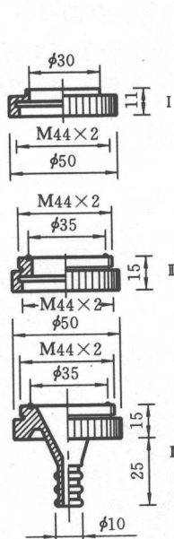
图 5 铝合金采样夹
