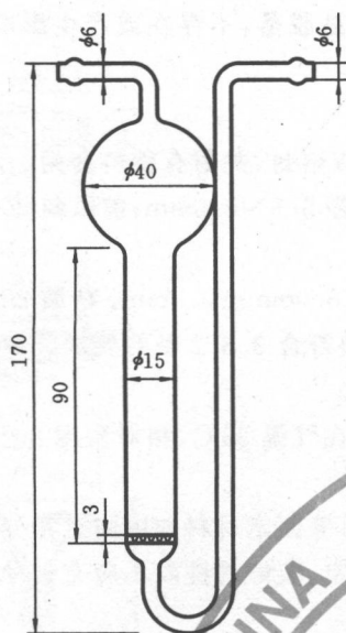
图 2 多孔玻璃吸收管
