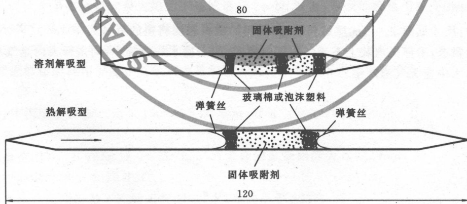
图 4 标准活性炭管和硅胶管
