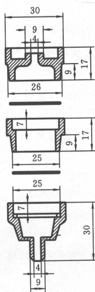
图 6 小型塑料采样夹
