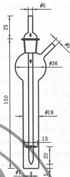
图 3 冲击式吸收管
